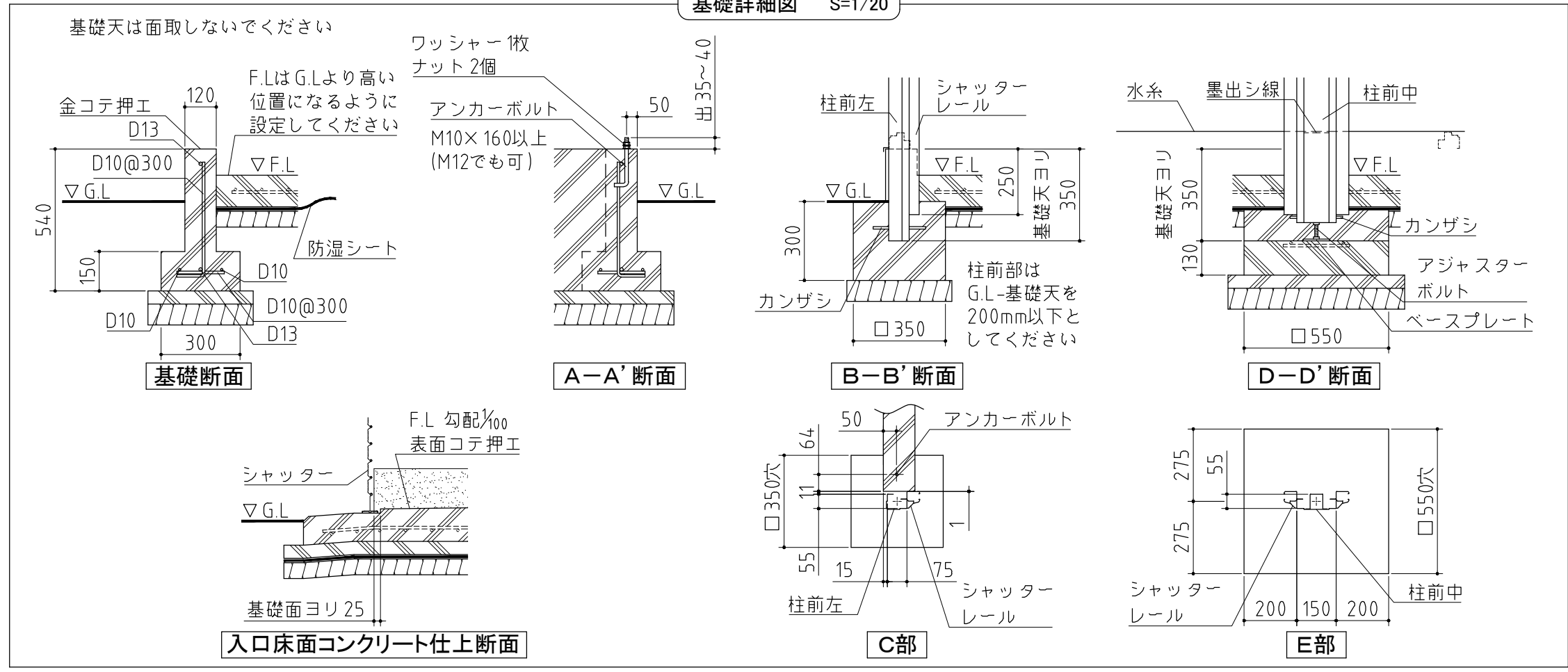
基礎詳細図 S=1/20
